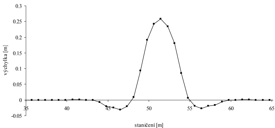
Obr. 8 Typický graf výchylky koleje s ocelovými Y-pražci po 600 mm (zde konkrétně pro spodní odhad příčné tuhosti a 100% odpor šterkového lože)
