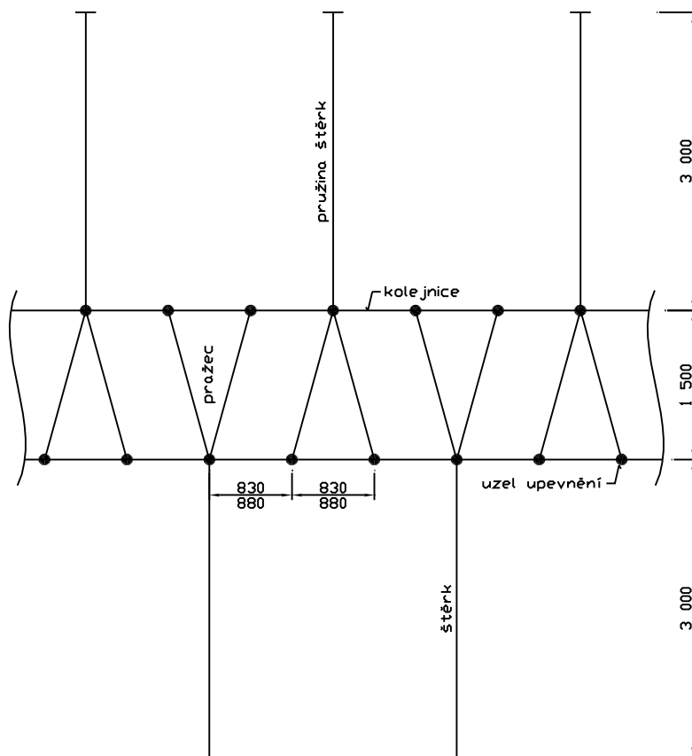
Obr. 6 Schéma diskrétního modelu koleje s ocelovými Y-pražci po 600 mm respektive 650 mm (vzdálenost uzlů upevnění 830 mm resp. 880 mm)
