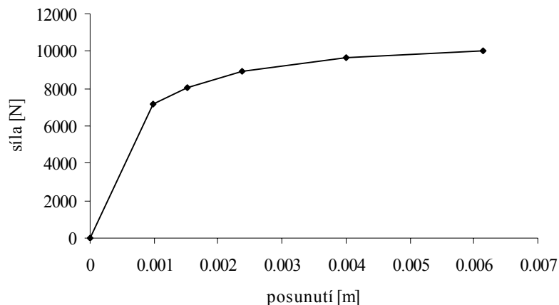
Obr. 3 Závislost síly na posunutí uvolněného betonového pražce kladeného po 600 mm ve šterkovém loži pro směr kolmo k ose kolejnice; převzato z [1]
