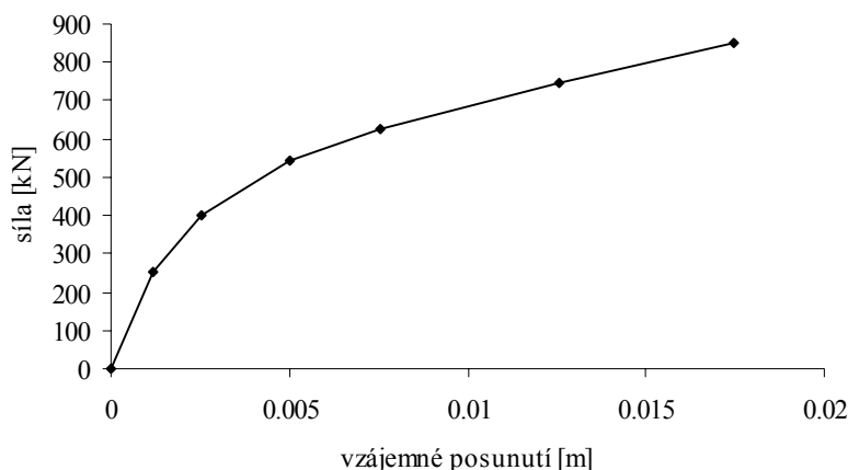
Obr. 2 Závislost síly na posunutí ve spoji kolejnice s pražcem pro posun kolmo k ose kolejnice (odpor k vzájemnému posunutí pražce a kolejnice v horizontální rovině); zjednodušeně přepočteno dle výrazu (1)
