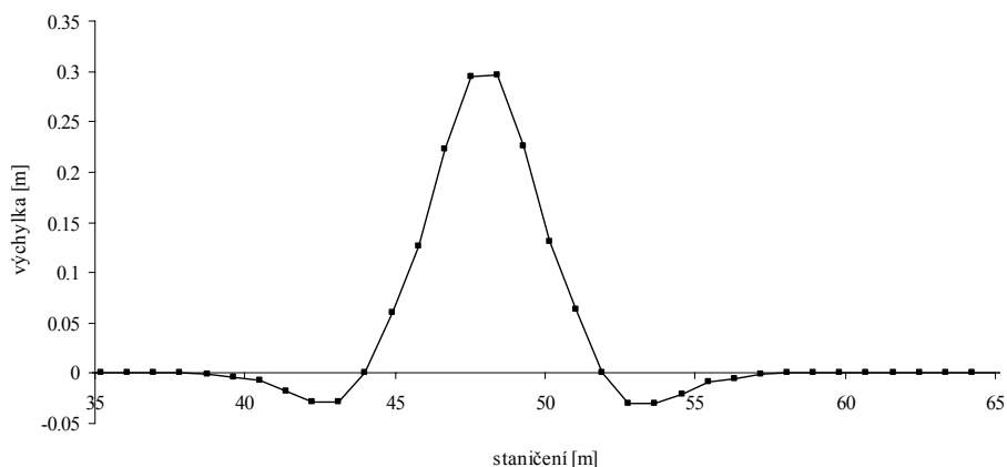
Obr. 9 Typický graf výchylky koleje s ocelovými Y-pražci po 650 mm (zde konkrétně pro spodní odhad příčné tuhosti a 100% odpor šterkového lože)
