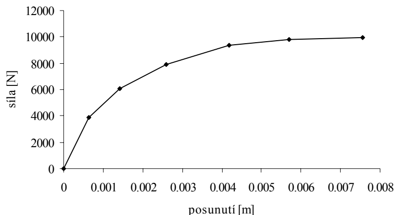
Obr. 4 Závislost síly na posunutí uvolněného ocelového Y-pražce kladeného po 650 mm ve šterkovém loži pro směr kolmo k ose kolejnice; převzato z [1]
