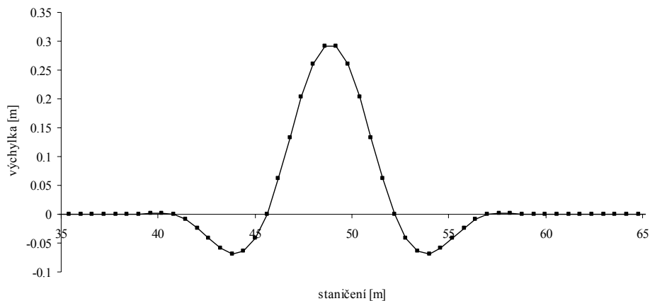
Obr. 7 Typický graf výchylky koleje s betonovými pražci po 600 mm (zde konkrétně pro horní odhad příčné tuhosti a 100% odpor šterkového lože)
