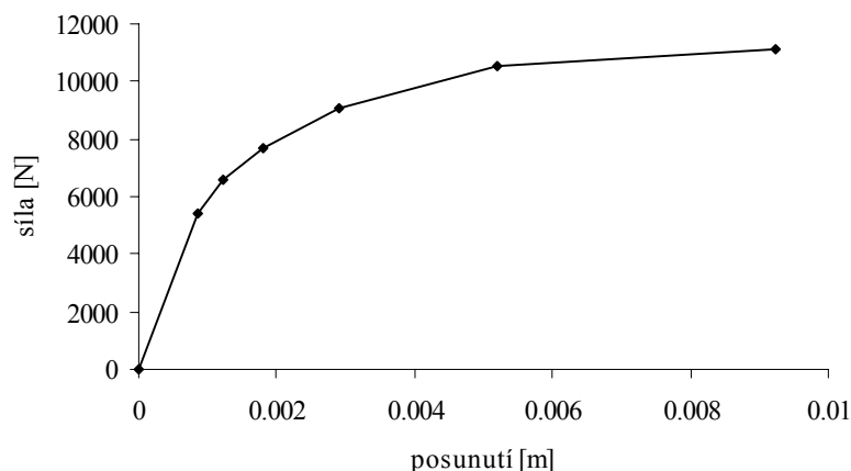
Obr. 4 Závislost síly na posunutí uvolněného ocelového Y-pražce kladeného po 600 mm ve šterkovém loži pro směr kolmo k ose kolejnice; převzato z [1]
