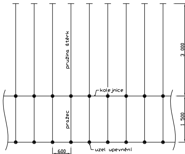
Obr. 5 Schéma diskrétního modelu koleje s betonovými pražci po 600 mm
