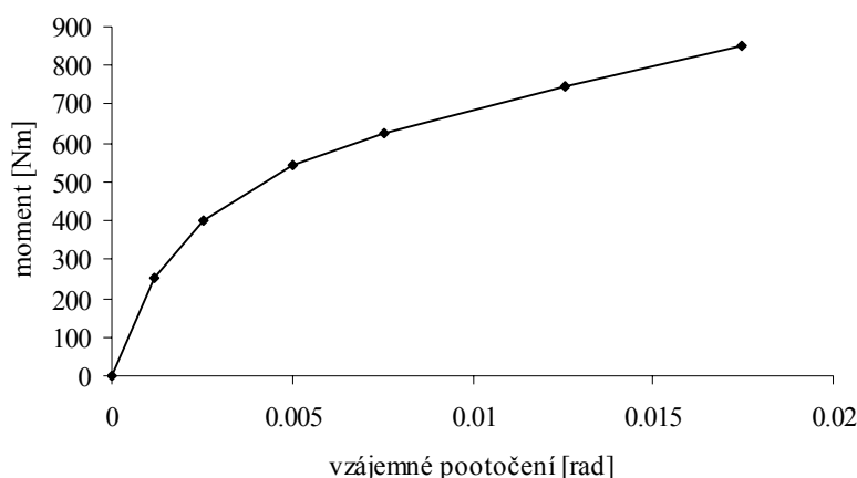
Obr. 1 Závislost momentu na pootočení ve spoji kolejnice s pražcem pro otáčení kolem vertikální osy (odpor k vzájemnému natočení pražce a kolejnice v horizontální rovině); převzato z [1]
